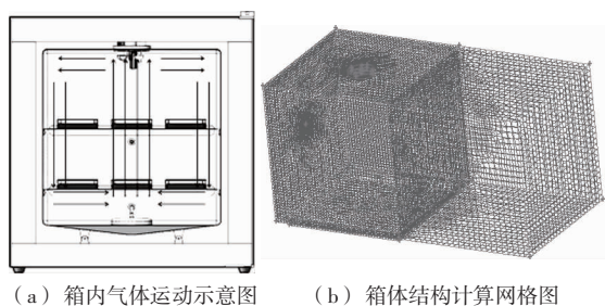
图1 箱体结构及箱内气体运动示意图
