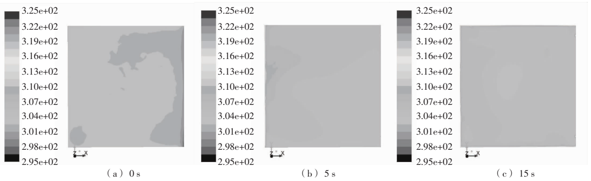
图 8 关门后 Z=0.23 m 截面的温度场(K)
