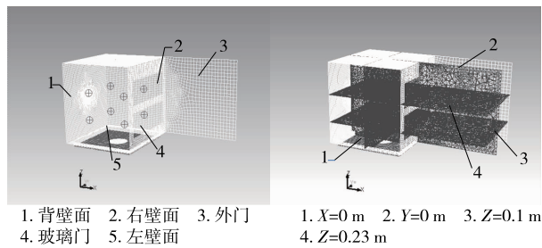
图2 物理模型监测点与监测面
