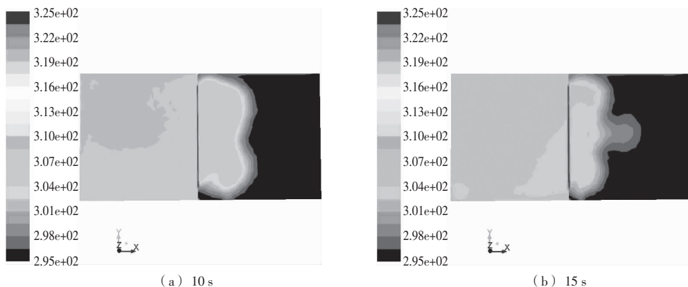
图6 开门后Z=0.23 m截面的温度场(K)
