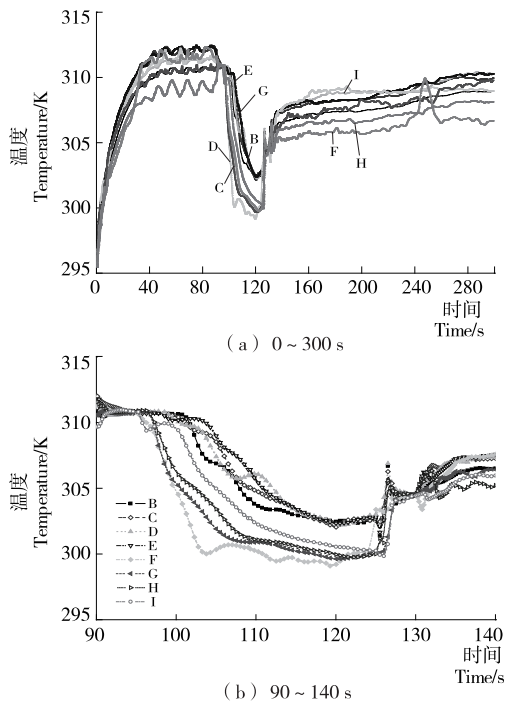
图 3 温度随时间变化曲线
