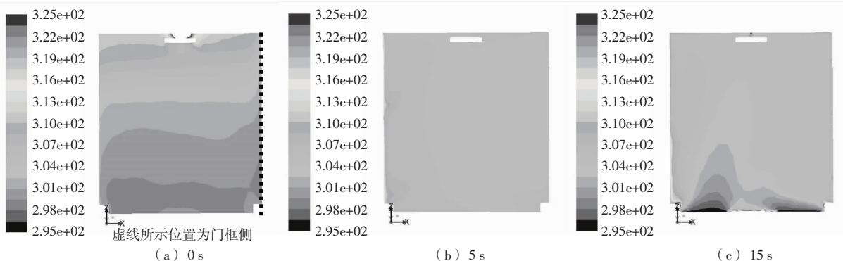
图7 关门后Y=0 m截面的温度场(K)
