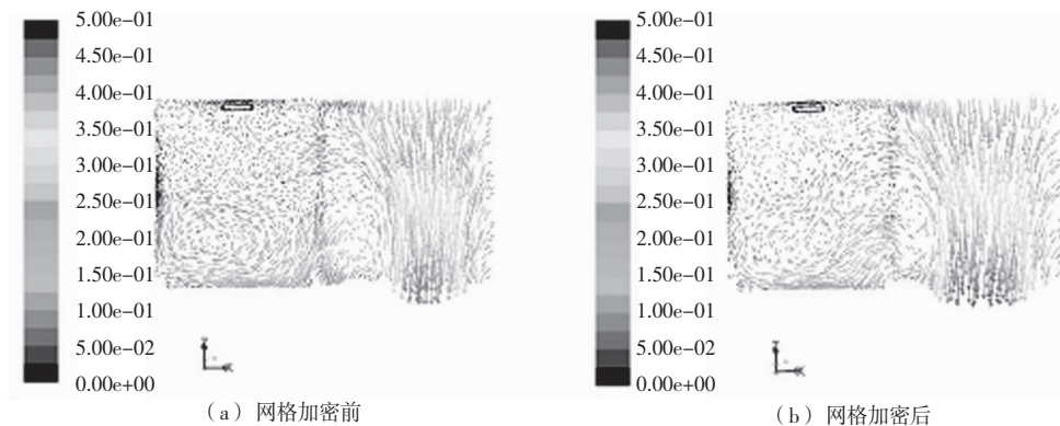
图5 开门10 s时Y=0 m截面的速度场(m/s)
