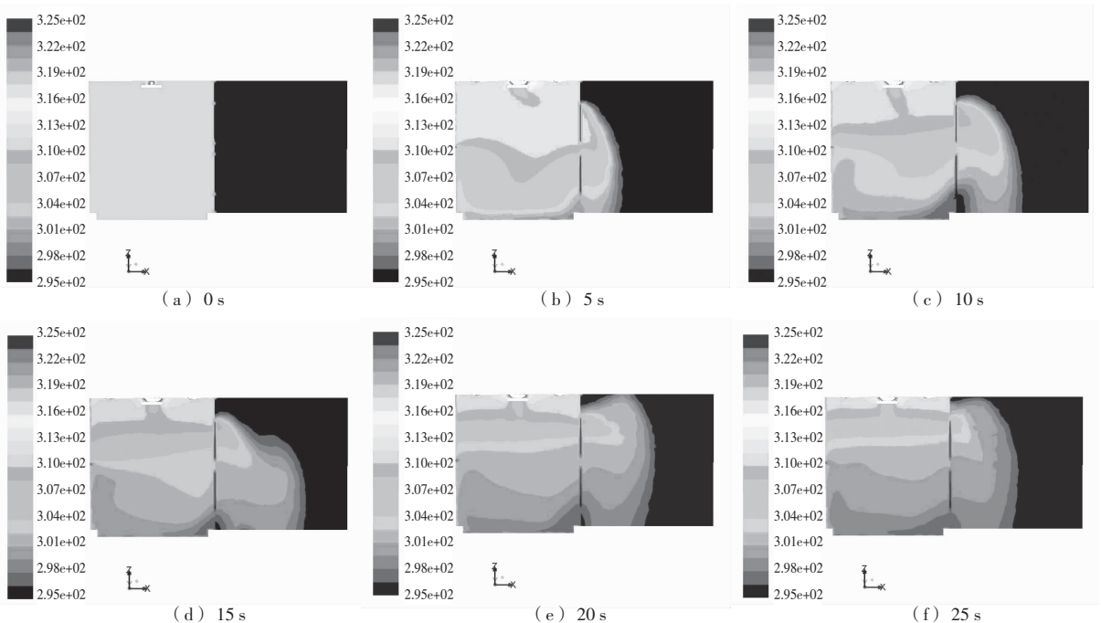
图 4 开门后 Y=0 m 截面的温度场(K)
