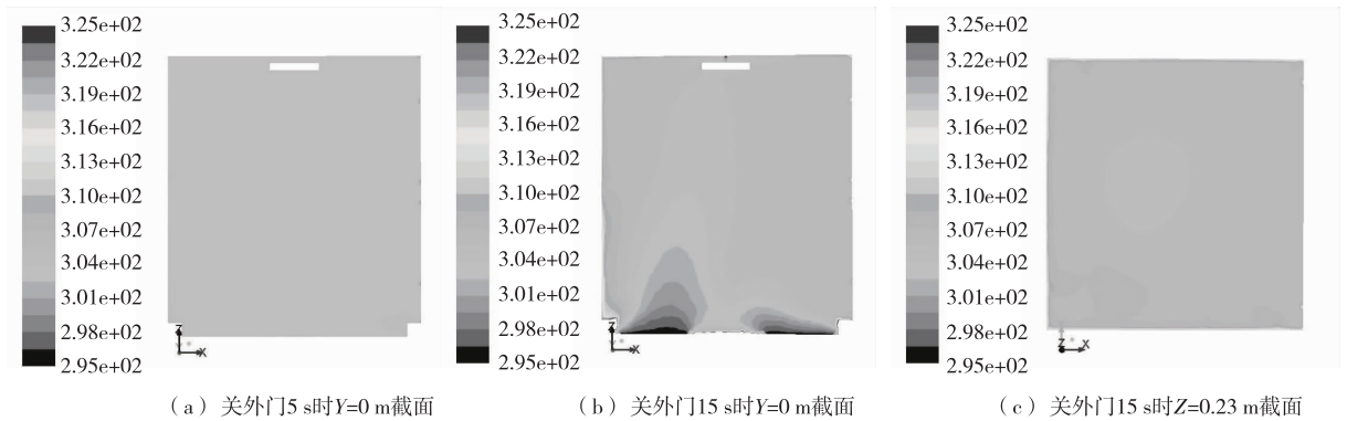
图 9 关门后的温度场优化分布
