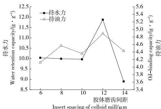
图 2 齿间距对 KPDP 持水力、持油力的影响
