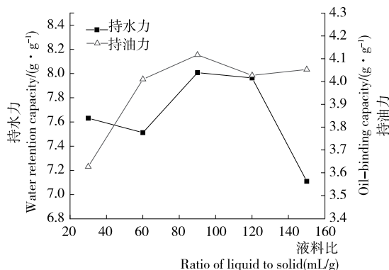
图 1 液料比对 KPDP 持水力、持油力的影响
